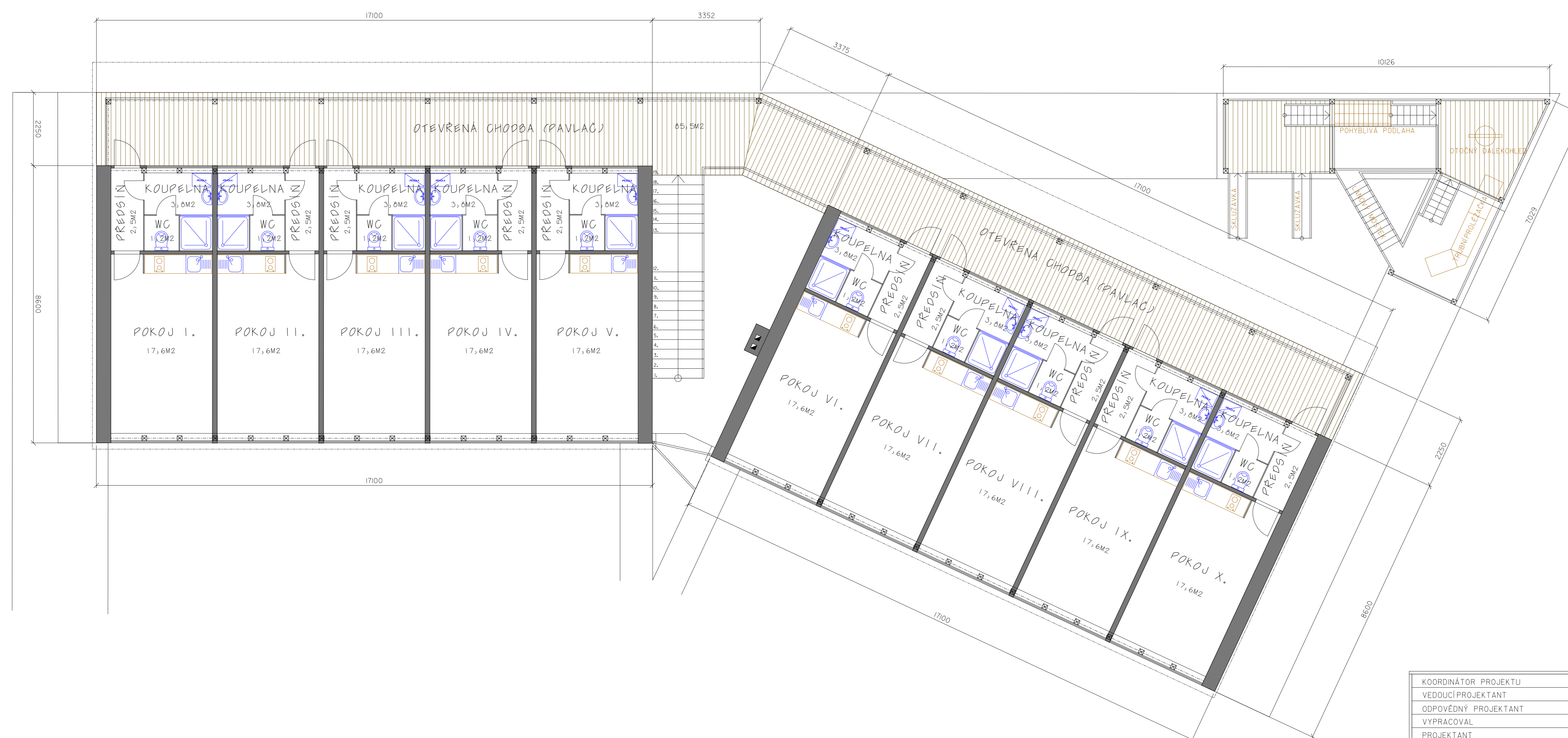
PŮDORYS 2. NP.
